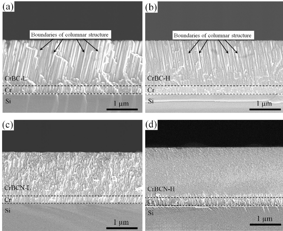
Fig. 3. Cross-sectional morphology of (a) CrBC-L (b) CrBC-H (c) CrBCN-L and (d) CrBCN-H coatings.
